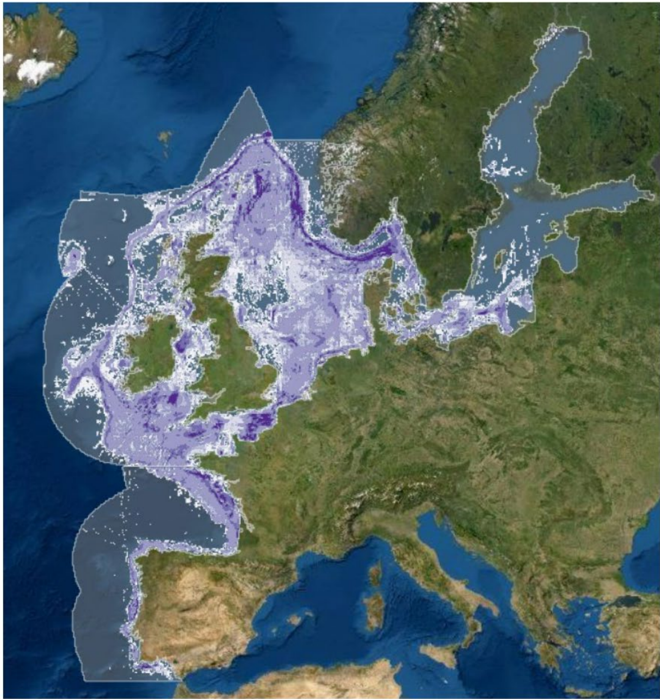
SAR (average 2013-2018)
